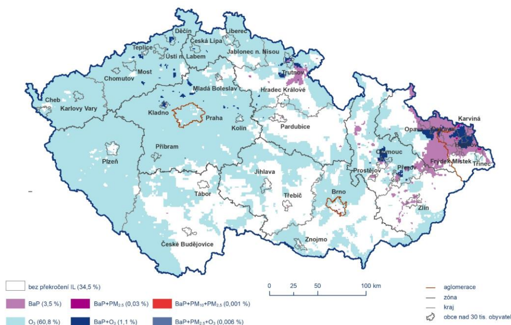
Obr. 2 Vyznačení oblastí s překročenými imisními limity pro ochranu zdraví vybraných skupin látek, 2020
