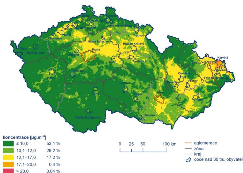
Obr. 5 Pole roční průměrné koncentrace PM 2,5 , 2020
