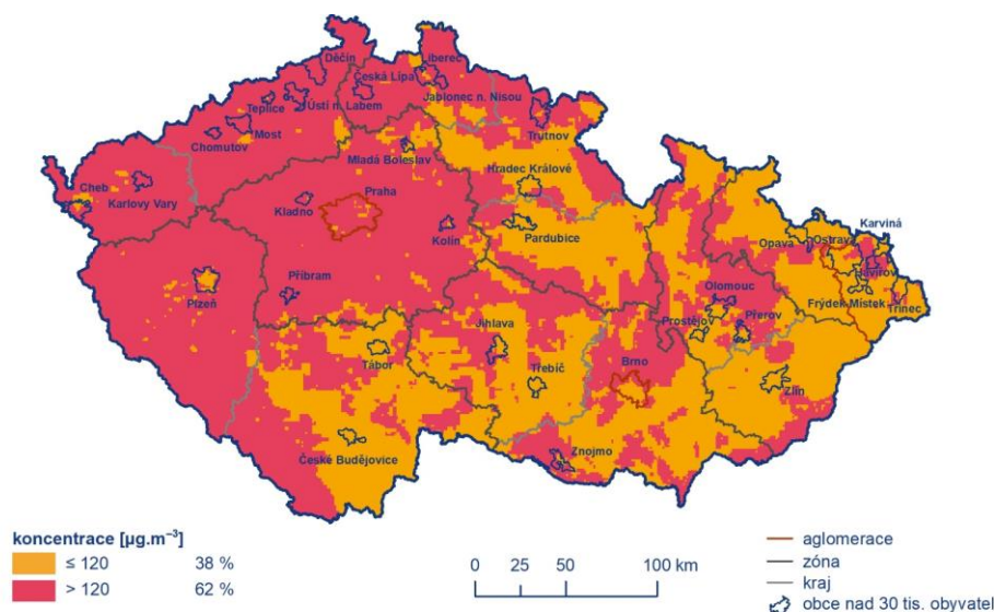
Obr. 7 Pole 26. nejvyššího maximálního denního 8hod. klouzavého průměru koncentrace přízemního ozonu v průměru za 3 roky, 2018–2020
