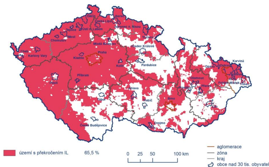
Obr. 4 Vyznačení oblastí s překročenými imisními limity pro ochranu zdraví se zahrnutím přízemního ozonu, 2020
