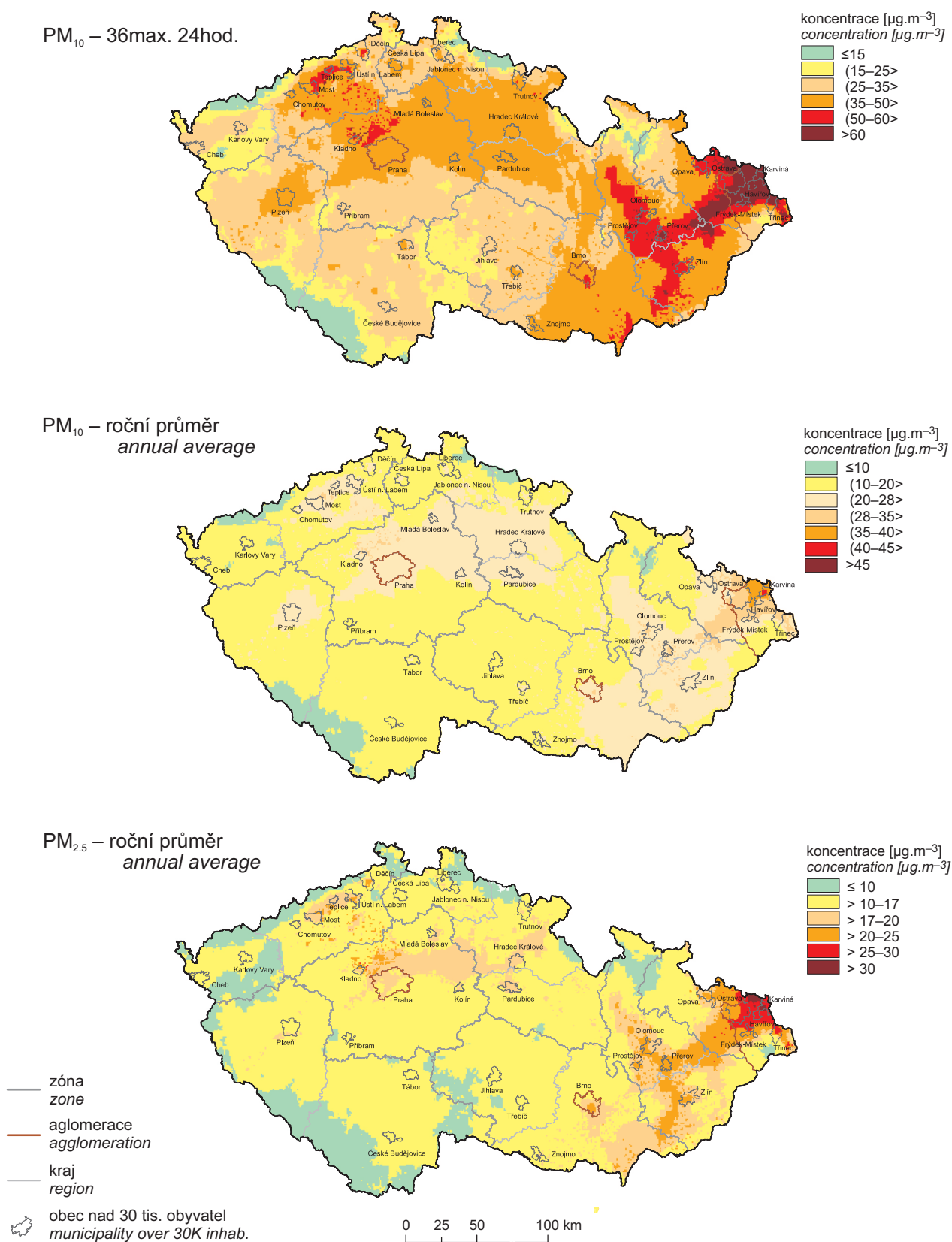
Obr. 1 Zobrazení plošných map pro PM 10 a PM 2.5 v barevné škále používané v Ročenkách znečištění ovzduší ČR do roku 2016
