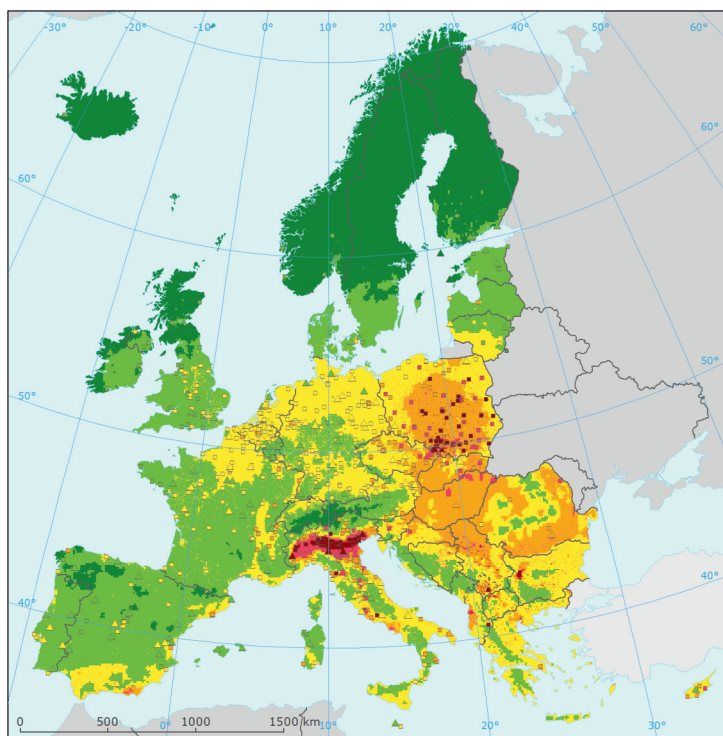
Obr. VIII.2 Průměrné roční koncentrace PM 2.5 v Evropě, 2015 Fig. VIII.2 Annual average concentration of PM 2.5 in Europe, 2015
