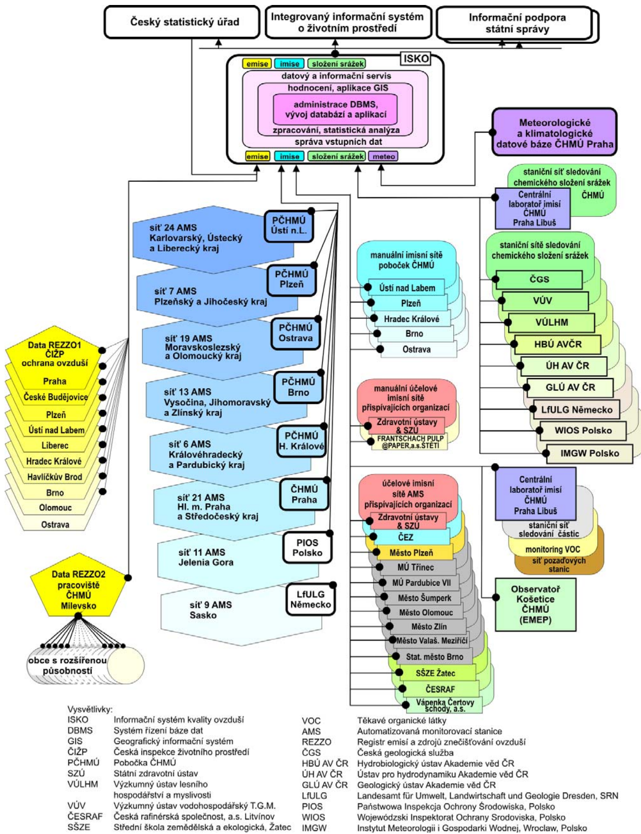
Obr. 1 Schema vazeb ISKO na zdroje dat a kooperující systémy v roce 2009
